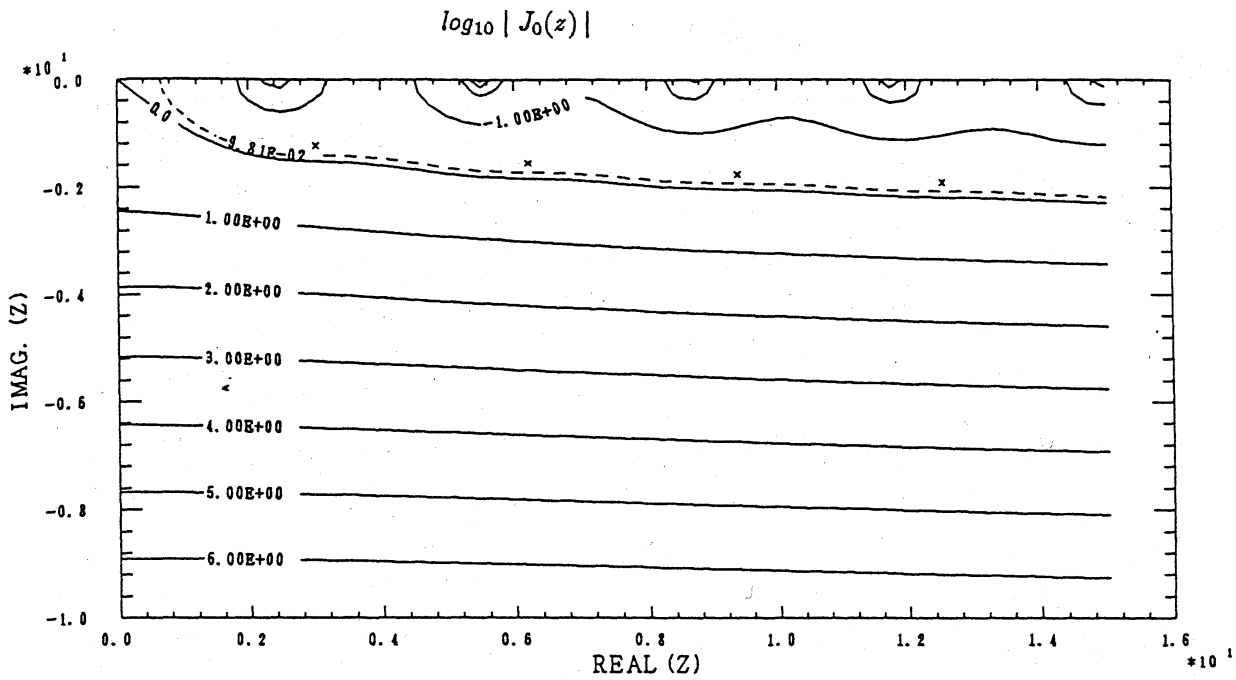
Fig.1 第 4 象限での \log_{10} |J_0(z)| の等高線 . x 印は J_0(z) - iJ_1(z) = 0 の根 ,
