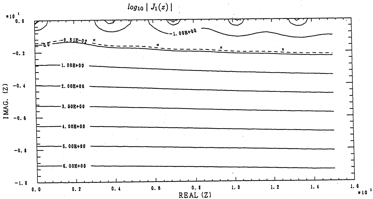
Fig.2 第 4 象限での \log_{10} |J_1(z)| の等高線 . x 印は J_0(z) - iJ_1(z) = 0 の根 ,
