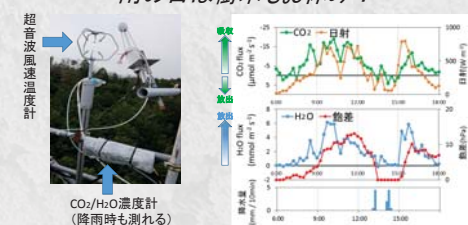
降雨終了後すぐにCO 2 吸収再開 雨滴の蒸発は空気が乾いてから
