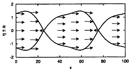
図 4.4: シート内の速度分布
