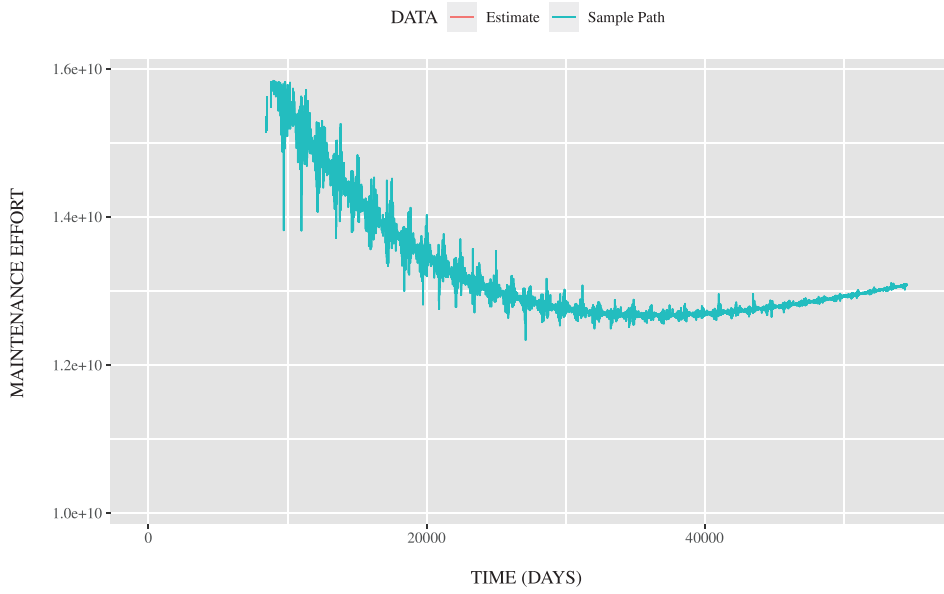
図 6 : \Lambda_{je}(t) の場合における推定された総開発工数 ( n = 3 ) .
