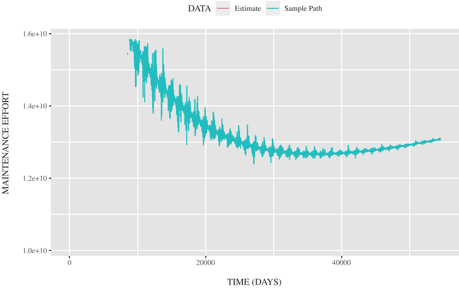
図 8 : \Lambda_{je}(t) の場合における推定された総開発工数 ( n = 5 ) .
