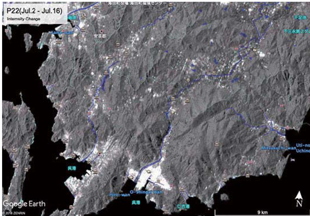
図-2（続き）．(c)南行軌道 P22 の広域観測モードの 2018 年 7 月 2 日と 16 日のペア．
