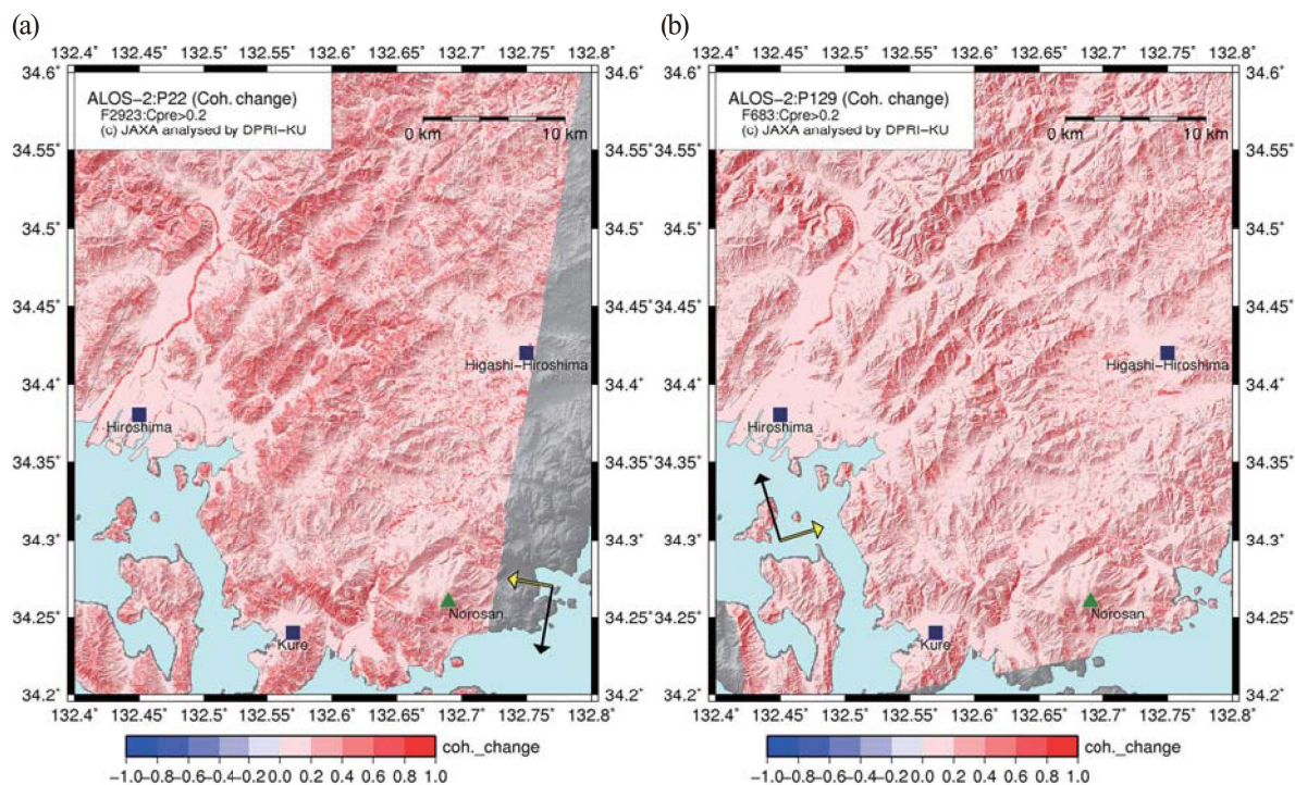
図-4. コヒーレンス変化. 災害前のペアのコヒーレンスが 0.2 以上の領域の \Delta\gamma . (a) 南行軌道 (P22). (b) 北行軌道 (P129).
