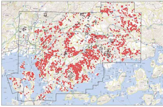
図-5. 国土地理院による航空写真判読から推定された崩壊地の分布 5)
