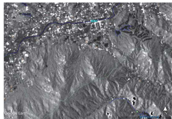
図-1. 強度画像の例。呉市～東広島市境界付近野呂山北麓の ALOS-2 強度画像。(a)2018 年 3 月 17 日、(b)2018 年 7 月 21 日。Google Earth により地理情報と重ね合わせた。
