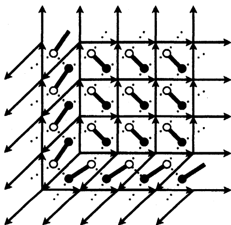
図 47: 「空の」ダイマー配置
