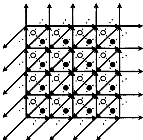
図 45: 普遍被覆
