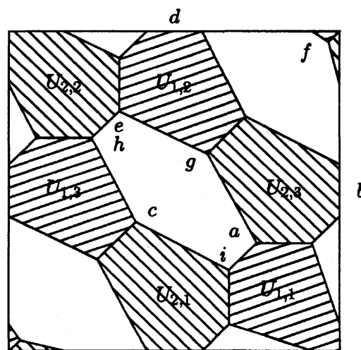
図 22: W_{\Delta_3}^{-1}(0) の形
