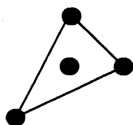
図 19: 三角形 \Delta_3
