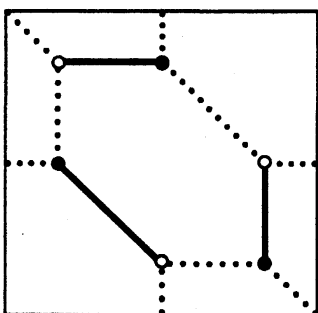
図 41: (h_x, h_y) = (0, 0)
