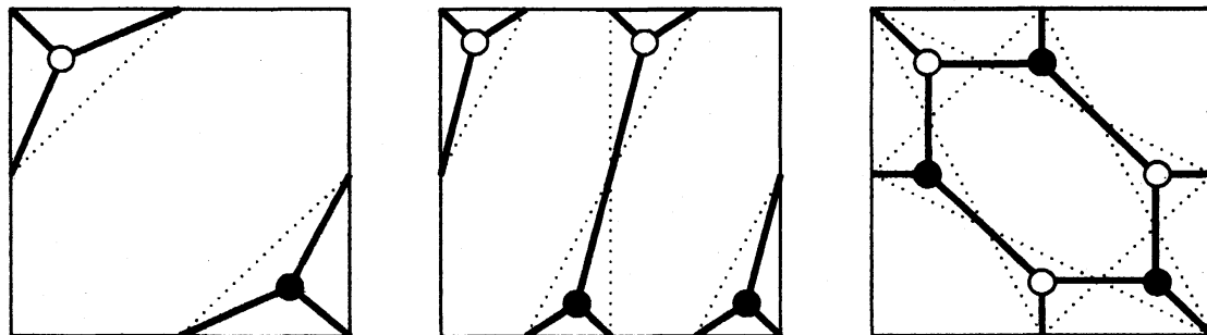
図 23: \Delta_1 に対応する 2 色グラフ 図 24: \Delta_2 に対応する 2 色グラフ 図 25: \Delta_3 に対応する 2 色グラフ
