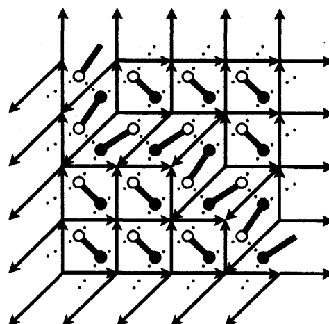
図 46: ダイマー配置と部分箭の関係
