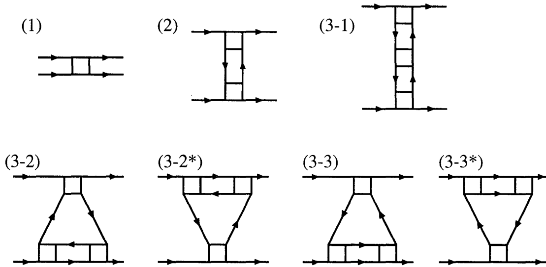
図 7: 既約 Vertex 関数の 3 次までの摂動項。実線は Green 関数 G_l^{(0)}(k) 、白抜き四角は裸の相互作用 I^{(0)} を表す。
