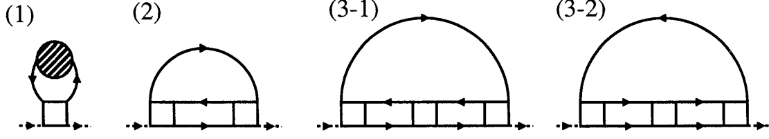
図 6: 正常自己エネルギー部分の 3 次までの摂動項。実線は Green 関数 G_\ell^{(0)}(k) 、白抜ききの四角は裸の相互作用 \Gamma^{(0)} を表す。(1) の斜線を施した円は、任意のダイアグラム構造を表す。
