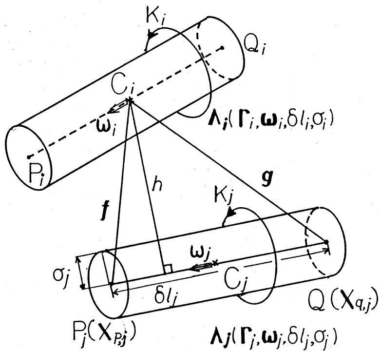
図. 3 要素の配置
