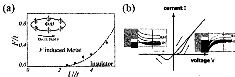
(a)モット絶縁体の臨界電場。 (b)モット転移を伴う強相関界面の IV 特性。
