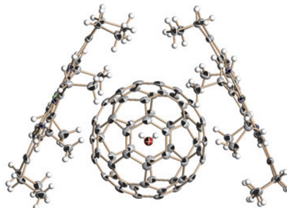
図2 2枚のポルフィリンに挟まれた \text{H}_2\text{O}@\text{C}_{60} の単結晶X線構造
