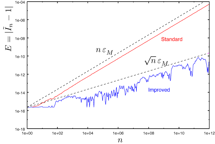
図 2: 式 (14) における不変量 \tilde{I}_n = \tilde{x}_n^2 + \tilde{y}_n^2 の変化
