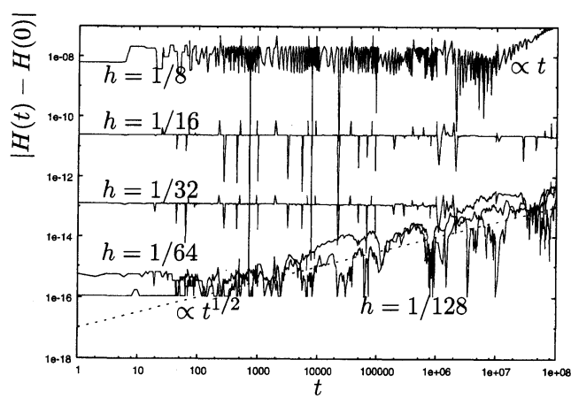
図 7: 4 段ガウス型 RK 法の実装法 (rkg44) におけるステップサイズ h と H の変化の関係
