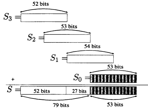
図 5: 三倍精度を用いた \sum_{j=1}^s a_{ij} f_j の計算
