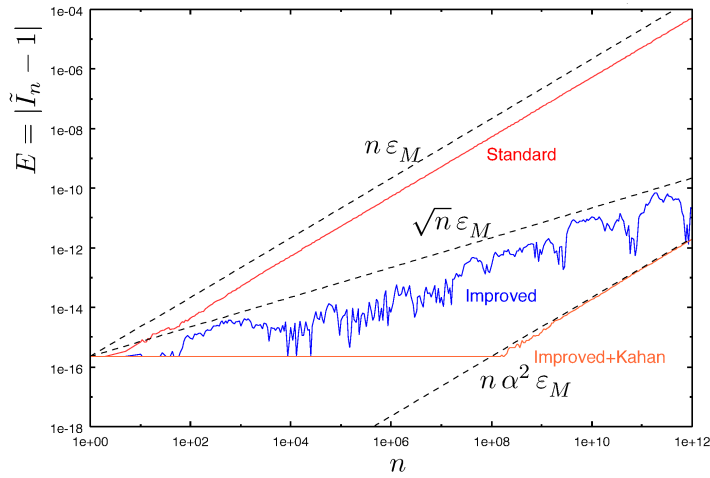
図 3: Kahan のアルゴリズムを用いたときの不変量 \tilde{I}_n = \tilde{x}_n^2 + \tilde{y}_n^2 の変化
