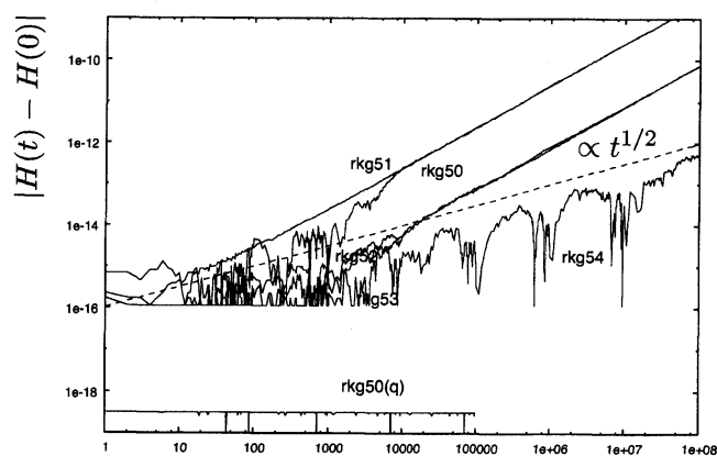
図 6: 5 段ガウス型 RK 法の 5 つの実装法の比較: Kepler 問題における H(q, p) の変化
