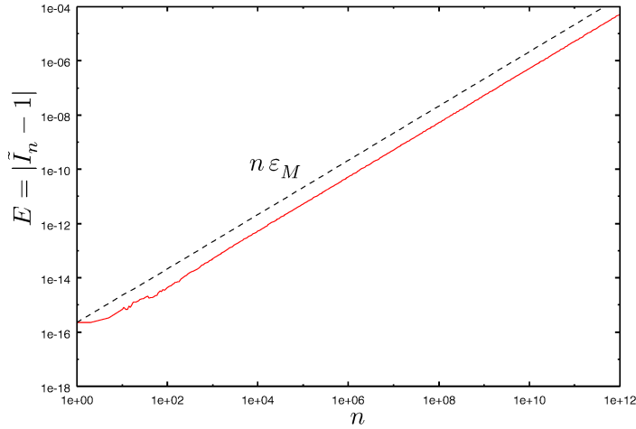
図 1: 式 (9) における不変量 \tilde{I}_n = \tilde{x}_n^2 + \tilde{y}_n^2 の誤差
