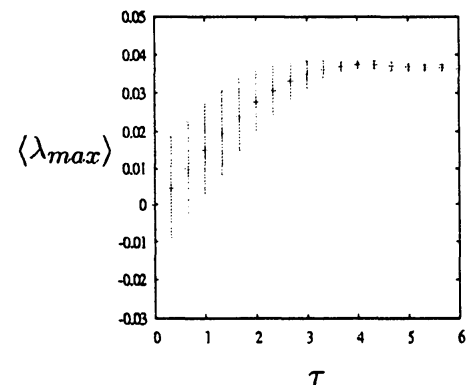
図 1 4 : 局所 Lyapunov 数[15]
