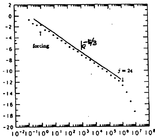
図 5 : エネルギースペクトル[9]
