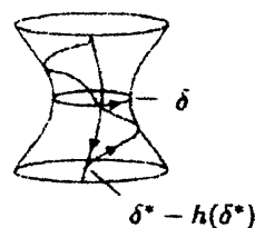
サイクル \delta^* - h(\delta^*)
