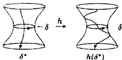
モノドロミー h の効果
