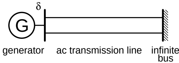
第1図 一機無限大母線系統. 1台の同期発電機が, 交流送電2回線を介して無限大母線(電圧・周波数不変の母線)に連系されている. 保護リレーは母線の直前に設置されている.
