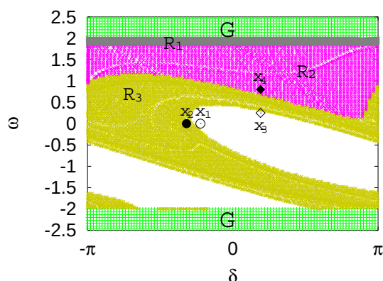
第3図 ハイブリッドオートマトンの可到達集合 ([23] から転載). 故障発生時 (時刻 0 s) における運転状態の集合 (初期状態の集合) である. G が危険集合, R_i (i=1,2,3) が可到達集合である. 添字 i は, 発電機が危険動作に至るタイミングを表している. 例えば, R_1 は離散値変数 q_1 で解軌道が危険集合 G に到達する, 即ち, 発電機が故障継続中に危険動作に至ることを表している.
