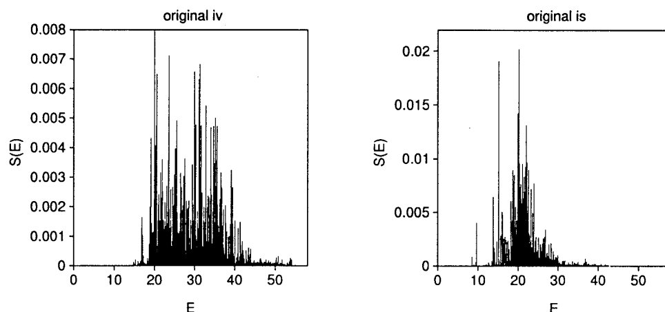
図3 ^{40}\text{Ca} 巨大四重極共鳴の理論計算による強度関数。左:アイソベクター型、右:アイソスカラー型。
