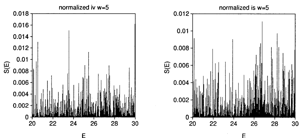
図4 normalize した強度関数 \bar{S}(E) 。左:アイソベクター型、右:アイソスカラー型。
