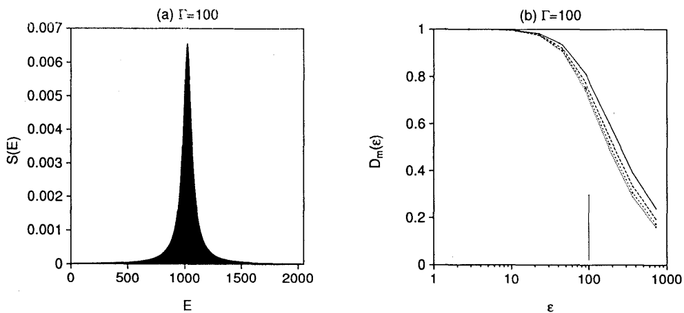
図 1 左：ローレンツ型強度関数、右：対応する局所スケーリング次元。上から D_m(\epsilon) ( m = 2, 3, 4, 5 ) を表す。
