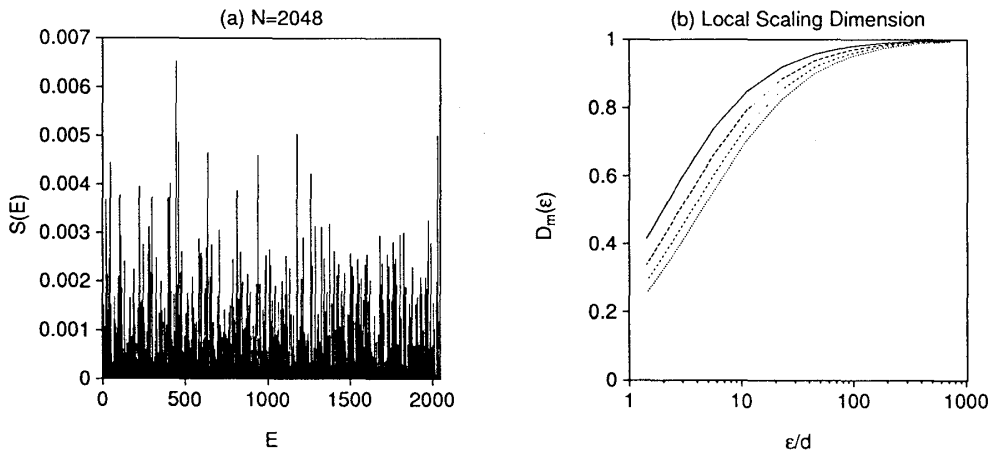
図 2 左：GOE から得られる強度関数の典型例、右：対応する局所スケーリング次元（アンサンブル平均の結果）。上から D_m(\epsilon) ( m = 2, 3, 4, 5 ) を表す。
