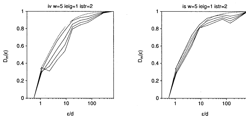
図5 局所スケーリング次元。左:アイソベクター、右:アイソスカラー。実線は上から D_m(\epsilon) ( m=2,3,4,5 ) を、点線は D_m^{\text{GOE}}(\epsilon) を表す
