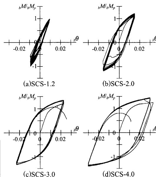
図2 復元力特性 (SCSシリーズ)
