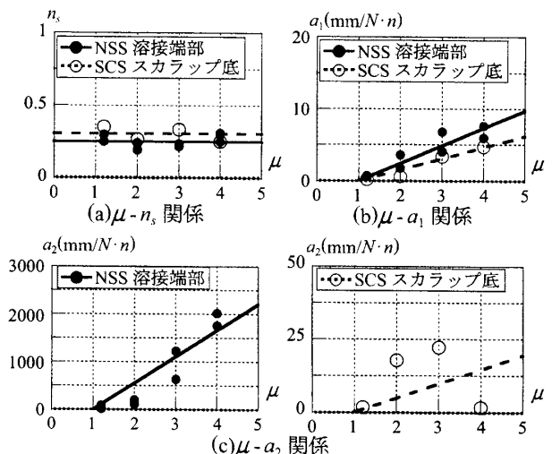
図8 亀裂進展に関する係数
