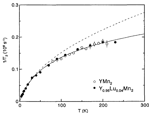
図 2: \text{Y}_{0.96}\text{Lu}_{0.04}\text{Mn}_2 および \text{YMn}_2 の ^{55}\text{Mn} の 1/T_2 の温度依存性。
