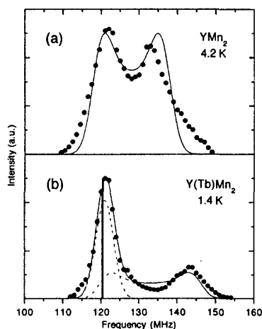
図 4: \text{YMn}_2 および \text{Y}_{0.97}\text{Tb}_{0.03}\text{Mn}_2 の磁気秩序状態の NMR スペクトル (補整済)。
