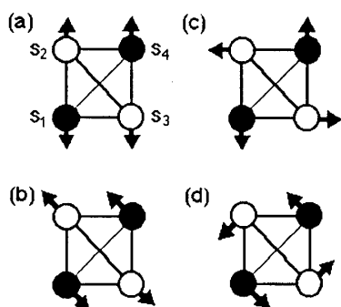
図 6: 単位四面体の 1\vec{q} 状態 (a)(b)、および 2\vec{q} 状態 (c)(d) の例。(●: z = 0 , ○: z = 1/4 )
