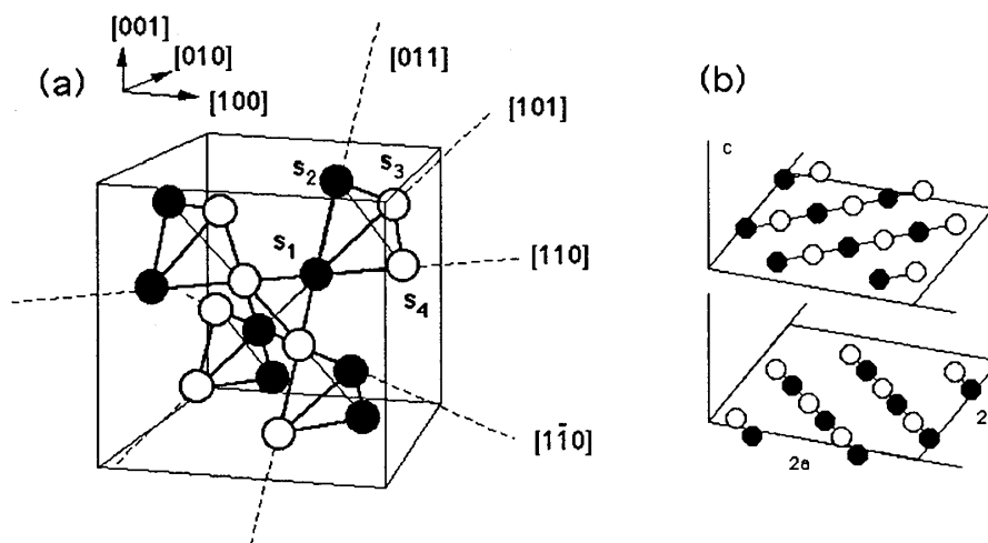
図 1: (a) 頂点共有四面体格子の黒白格子の一例。(b) c 面の配列を強調したもの。
