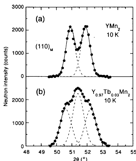
図 3: \text{YMn}_2 および \text{Y}_{0.97}\text{Tb}_{0.03}\text{Mn}_2 の (110) 磁気ブラッグピーク。
