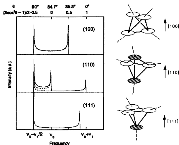
図 5: スピン回転面が \{100\} , \{110\} , \{111\} のときに期待される NMR スペクトル。右側の図はそれぞれの場合の局所対称軸 (点線) とスピン回転面 (楕円) との関係を示す。白抜きの楕円と斜線をかけた楕円は対称軸と回転面の相対関係が異なるものを示す。
