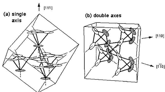
図 7: \text{Y(Tb)Mn}_2 の1軸ヘリカル構造と2軸ヘリカル構造の略図。楕円はスピン回転面を、点線は局所対称軸を表す。白い楕円と斜線をかけた楕円は、スピン回転面と対称軸との関係が異なるものを表す。
