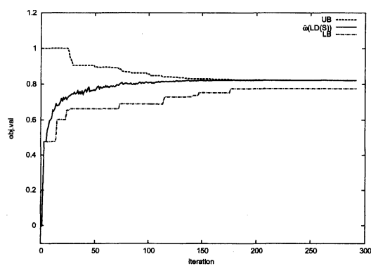
图 6: s838
