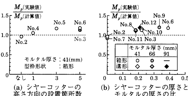
図 2 全塑性曲げ耐力に及ぼすシヤーコッターの影響
