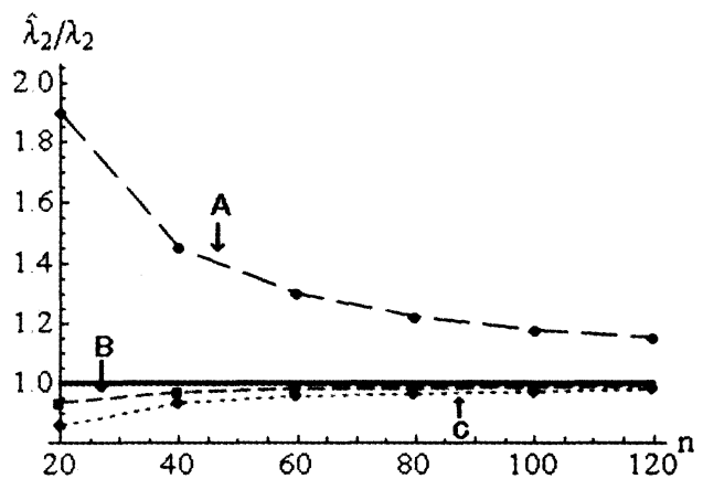
図 1-2. 第 2 固有値
