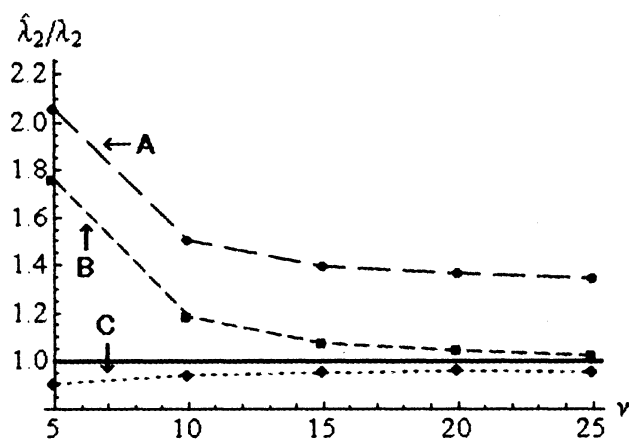
図 4-2. 第 2 固有値
