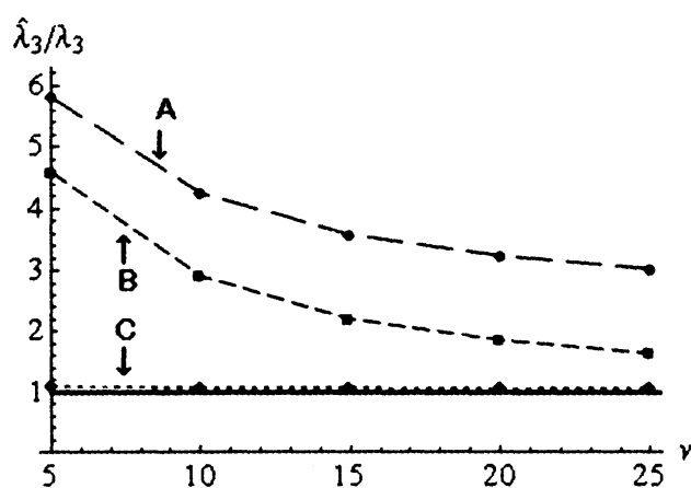
図 4-3. 第 3 固有値
