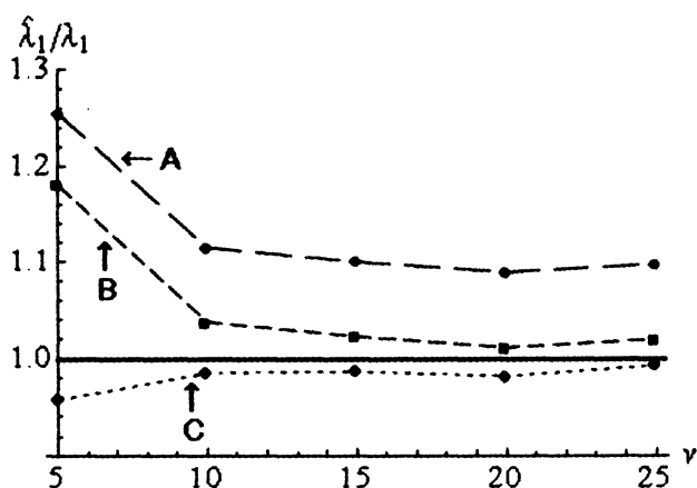
図 4-1. 第 1 固有値
