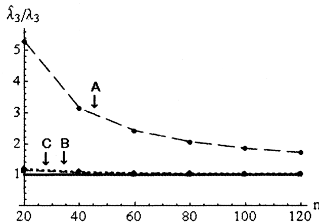
図 1-3. 第 3 固有値
