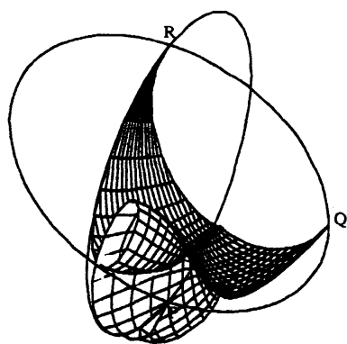
X の上半分の像
