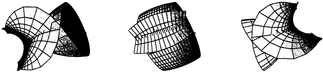
図 3: 又黒による X^\circ の像
