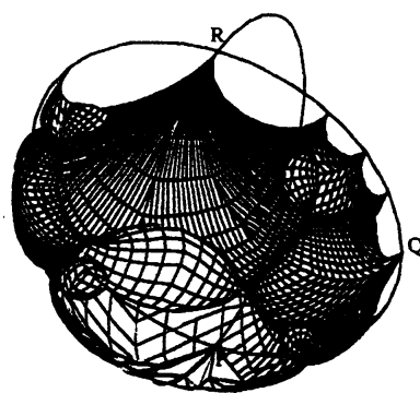
上下合わせて10半平面の像
