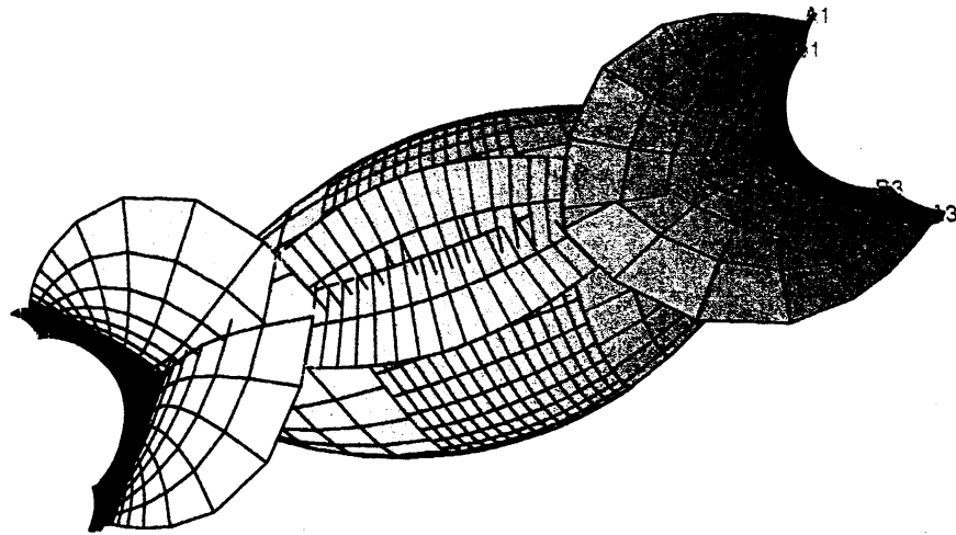
図 3: 又黒による X^\circ の像
