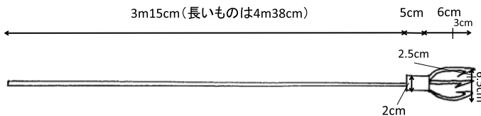
図 16 大型の鉈サパーの一例
