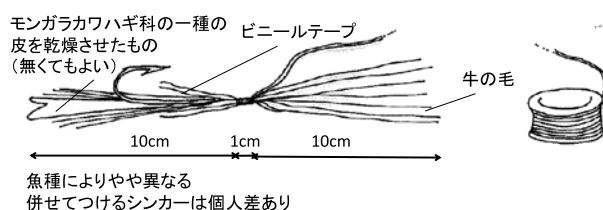
図 7 牛の毛やモンガラカワハギ科の魚の皮を利用した疑似餌釣り漁具マンチョーの一例
