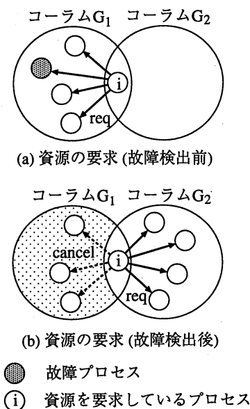
図 1 資源の要求メッセージの取消
