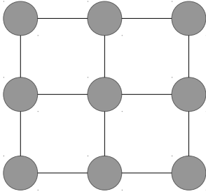
図 1 格子型グラフの例
