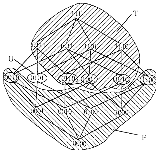
図3 例3.1の部分関数 g
