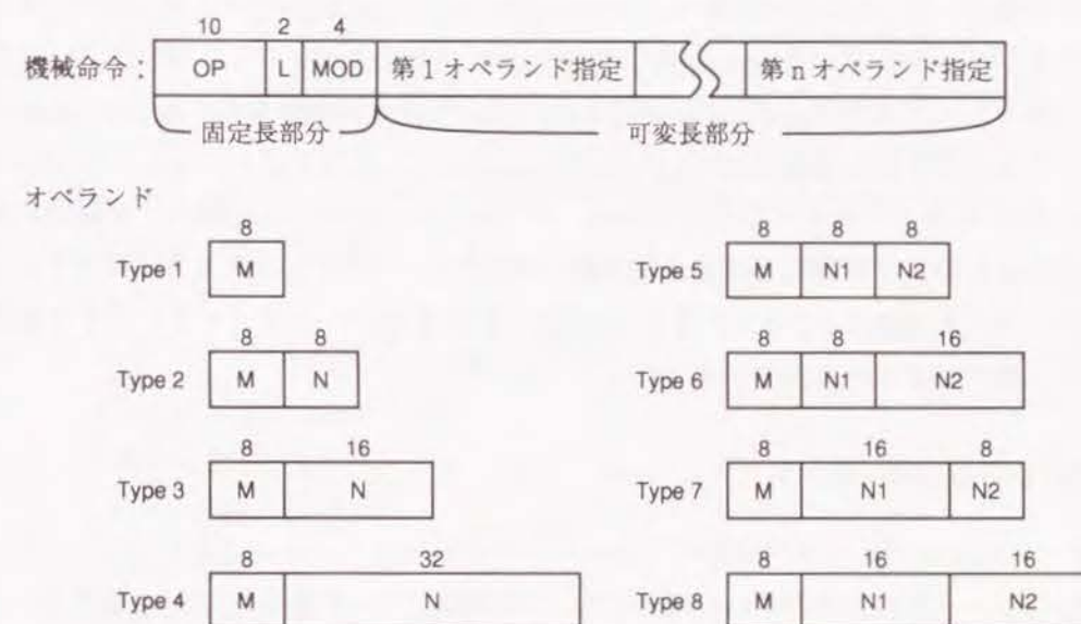
図 6.5: 機械命令の形式
