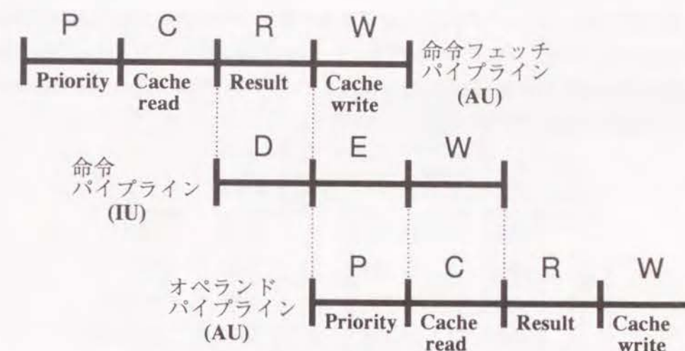
図 9.7: 命令フェッチ/オペランドパイプライン
