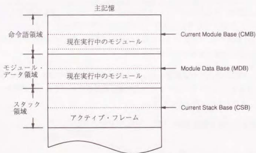
図 6.4: 主記憶の構成
