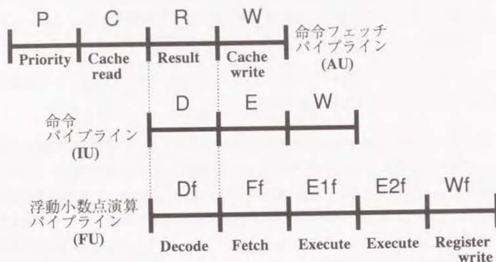
図 9.6: 浮動小数点演算パイプライン
