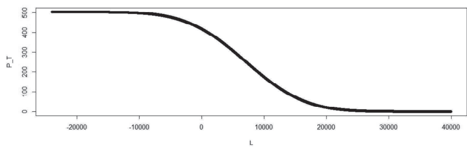
図 1：業績条件 L を-24,000 から 40,000 まで変化させたときの P_T のプロット結果
