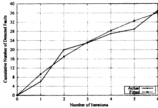
図 2: 推定された平均値関数 \hat{H}_n
