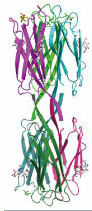
図:SLL-2と糖の複合体構造
