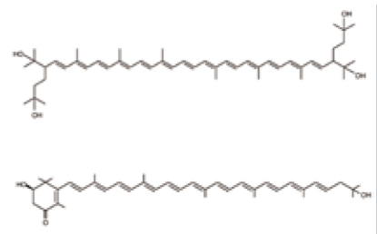
図:代表的な放射線耐性細菌 Rubrobacter radiotolerans (上)、 Deinococcus radiodurans (下)の含有赤色カロテノイド色素の構造
