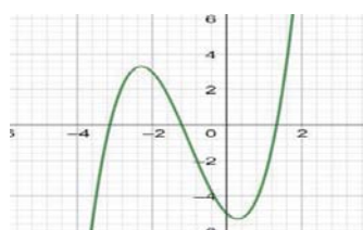
f(x) = x^3 + 3x^2 - 2x - 5 のグラフ
