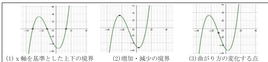
f(x) = x^3 + 3x^2 - 2x - 5 のグラフ
