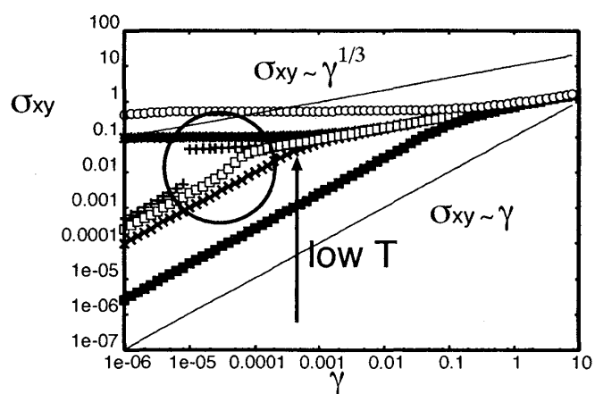
Figure 2: 式 (1) で記述される、 \sigma_{xy} の \gamma 依存性。
