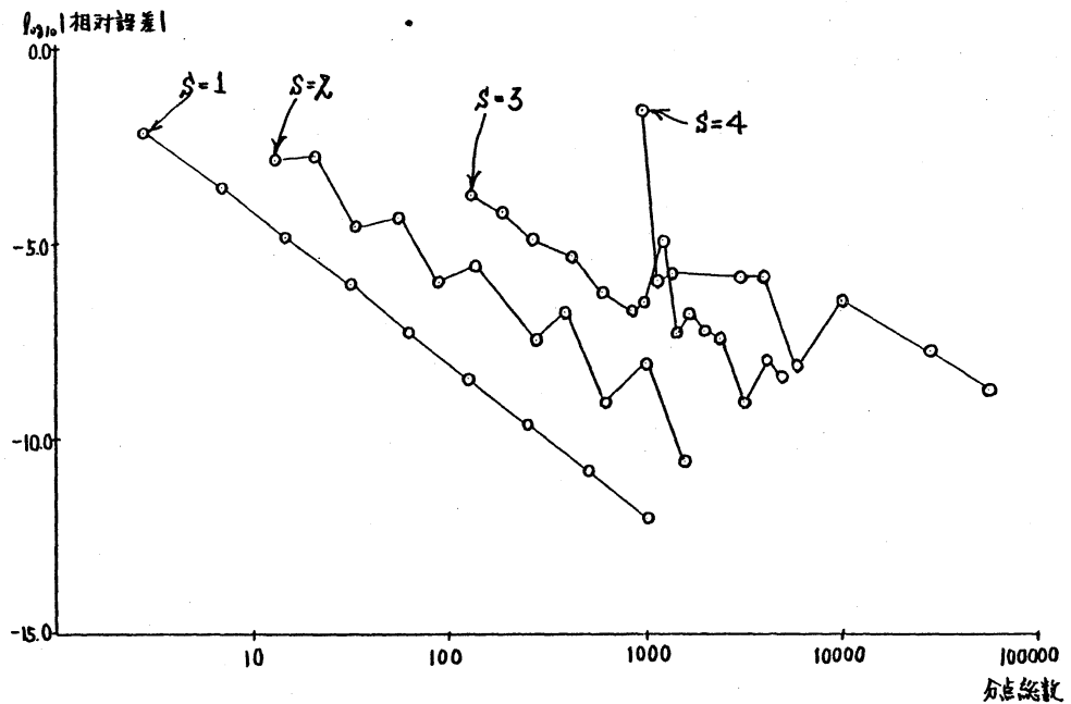
图4. 积分问题 \int_{[0,1]^s} \prod_{j=1}^s \exp(x_j)/x_j dx 多项式变换 ( k=5 ) + good lattice points 法通用 L_N 时的相对误差.
