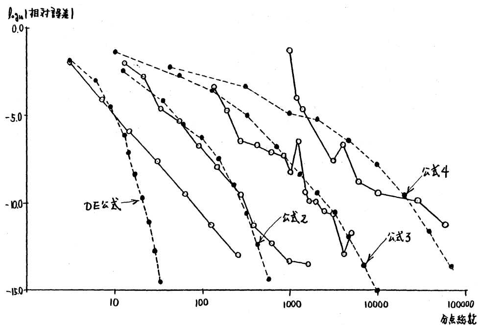
図7. 積分問題 \int_{[0,1]^s} \prod_{j=1}^s \exp(x_j) dx に DE公式, 公式2~4 を適用 ( k 時の相対誤差. (○は good lattice points 法の結果))
