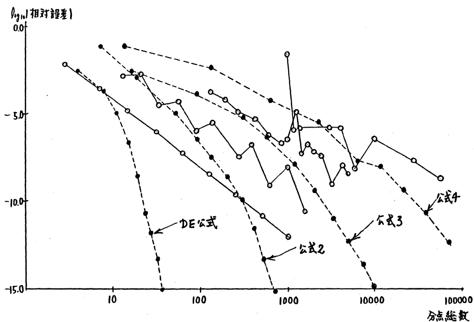
図8. 積分問題 \int_{[0,1]^s} \prod_{j=1}^s \exp(x_j)/x_j dx に DE公式, 公式2~4 を適用 ( k 時の相対誤差 (○は, good lattice points 法の結果))
