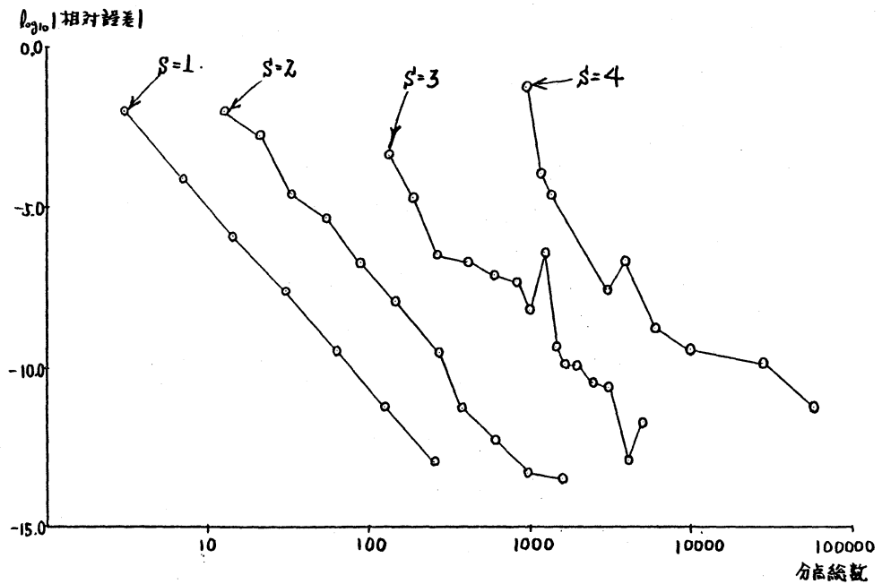
图3. 积分问题 \int_{[0,1]^s} \prod_{j=1}^s \exp(x_j) dx 多项式变换 ( k=5 ) + good lattice points 法通用 L_N 时的相对误差.
