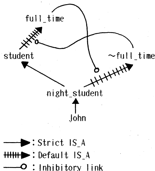
図2 ネットワーク表現
