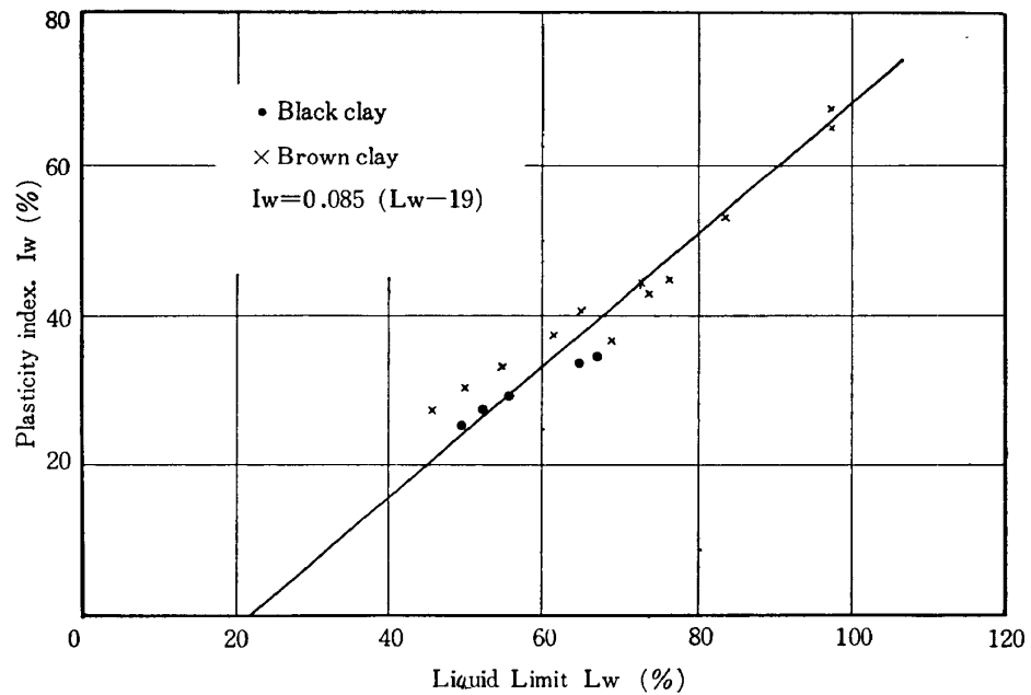
図-9 土のコンシステンシー 土質改良のための身長測定
