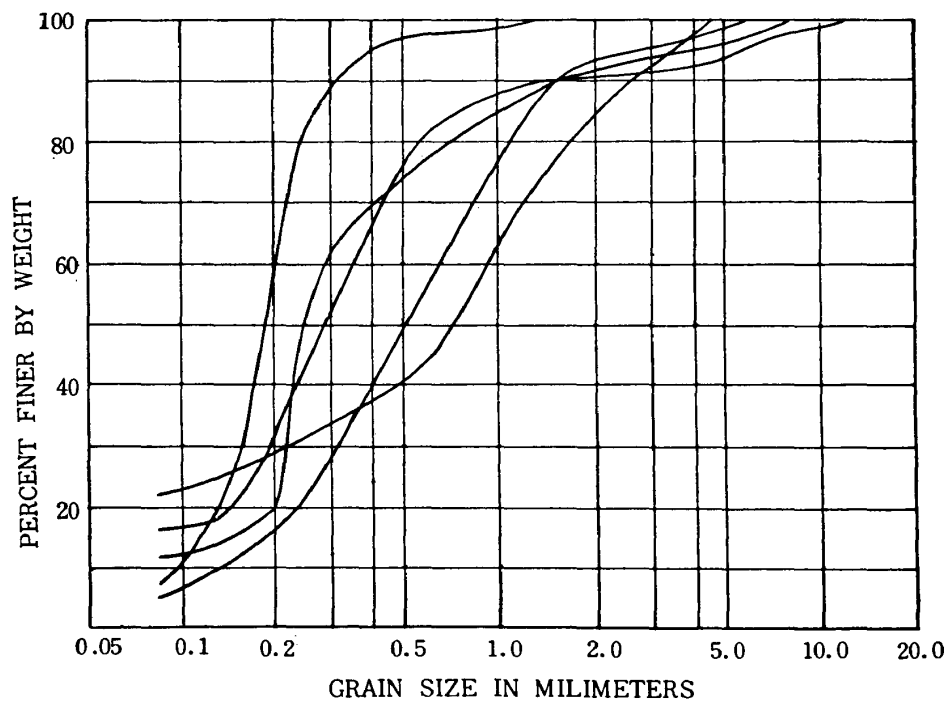
図-8 粒 度 分 布
