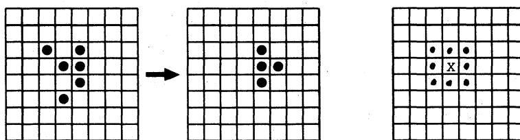
図 1: ライフゲームの例 と セル x の周りの 8 個のセル
