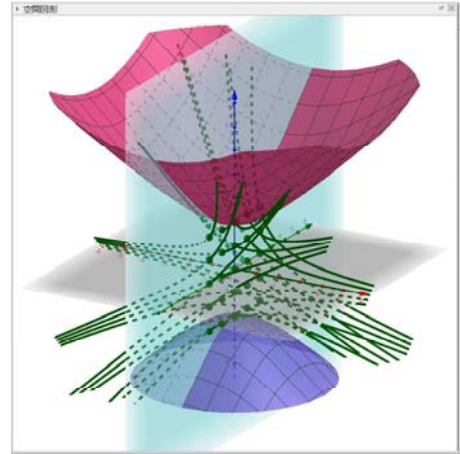
図 5: 対角行列による左移動のフロー
