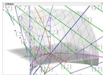
図 3: “ d = 1 ” 曲面
