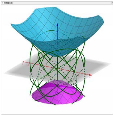
図 4: 回転行列による左移動のフロー
