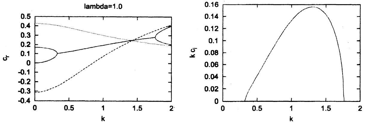
図 6: 左: \lambda = 1.0 での分散曲線 (実線). 右: 擾乱の成長率. 破線, 点線はそれぞれ部分系 (30), (31) の分散曲線.
