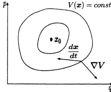
図 2: 2次元の力学系. \dot{V} = dV/dt \leq 0 であり, かつ \mathbf{x} = \mathbf{x}_0 で V(\mathbf{x}) は極小値となる.
