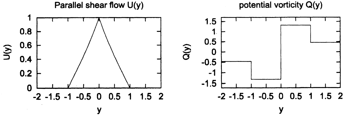
図 4: 左: \lambda = 1.0 での (27). 右: \lambda = 1.0 での (29).
