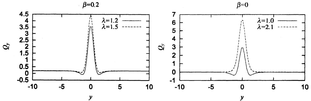
図 3: 左: \beta = 0.2 , \lambda = 1.2, 1.5 での Q_y . 右: \beta = 0 , \lambda = 1.0, 2.1 での Q_y .
