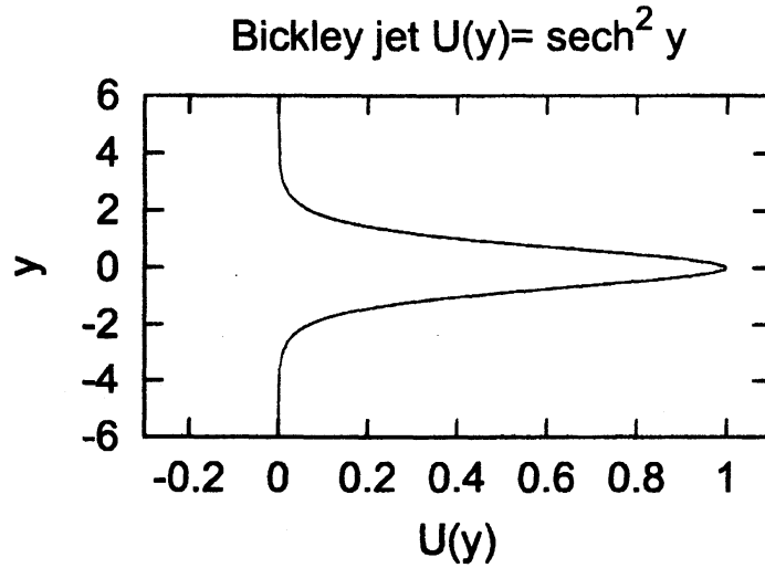
図 1: 速度場 U(y) = \text{sech}^2 y .
