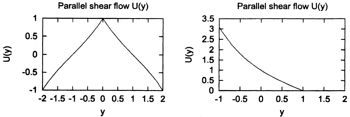
図 5: 左: \lambda = 1.0 での (30). 右: \lambda = 1.0 での (31).
