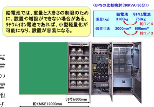
図.1 鉛電池とリチウムイオン電池の
