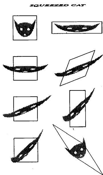
図 6: ローレンツ変換による回転
