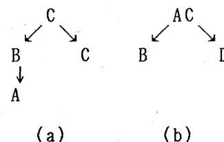
図2 関数従属性の反映
