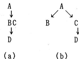
図3 多値従属性の反映
