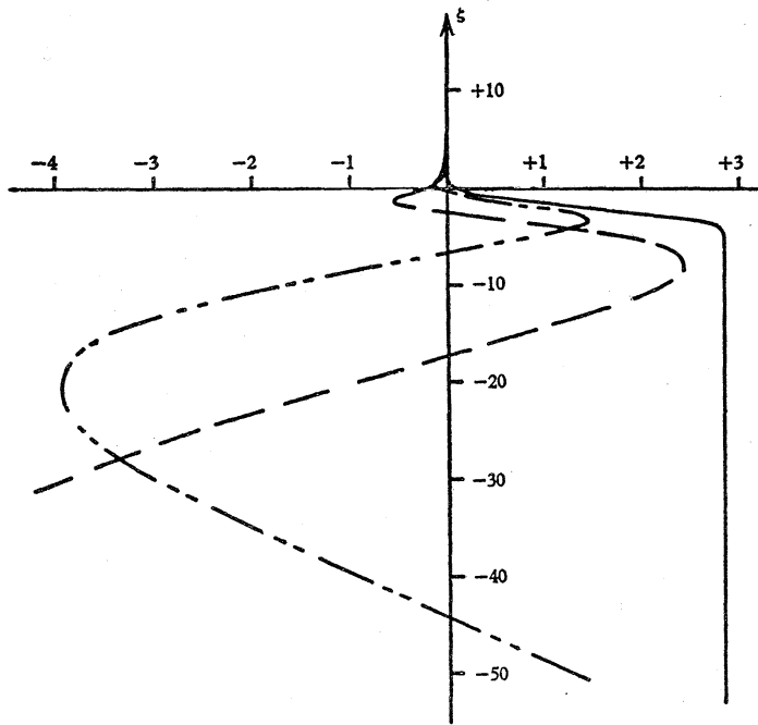
第3図 実線 = レイノルズ応力 鎖線 = w の虚数部 2本鎖線 = w の実数部
