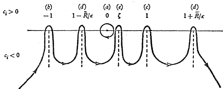
図21 図 ラプラス逆変換式 (3-19) における \gamma > 0 の場合の積分路
