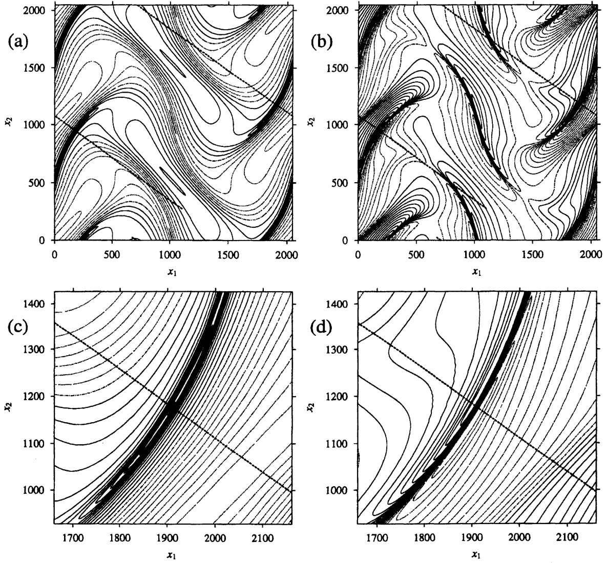
図 1: (a) para-real 平面 \mathbf{y} = (2\pi/64)(\cos(-\pi/6), \sin(-\pi/6)) での時刻 t = 1.65 における渦度の実部の等高線。実線は負、一点鎖線はゼロ、点線は正の値をあらわし、等高線間隔は 1.0。格子点数は 2048^2 で para-real 平面全体を表示している ( \mathbf{y} を固定して 2\pi 周期の (x_1, x_2) 平面で見ている)。(b) 渦度の虚部の等高線。パラメータは (a) と同じだが、等高線間隔は 0.2。(c) 渦度の実部の等高線。特異的な振舞いをしている点 (複素渦度の大きさ \sqrt{\omega_r^2 + \omega_i^2} が最大となる点) 付近を拡大したもの。(d) 渦度の虚部の等高線。特異的な振舞いをしている点付近を拡大したもの。
