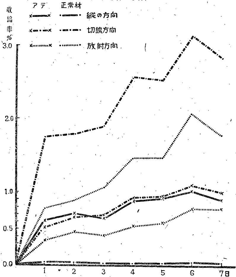
第15図 アカマツ材の室内乾燥によるアテと正常材の収縮速度比較 (11月1日—8日)
