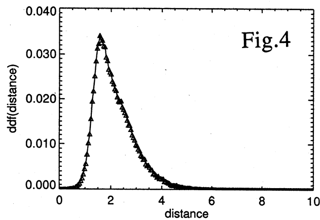
図 4 “ソリトン”間の間隔分布（計数の閾値 \Delta = 0.5 ）
