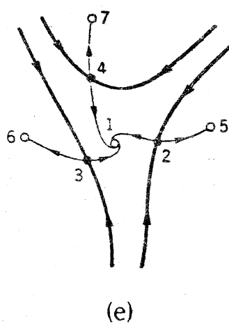
図4 (4)式の変換 T による不動点・同期点と不変曲線
