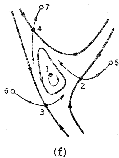
図4 (4)式の変換 T による不動点・同期点と不変曲線
