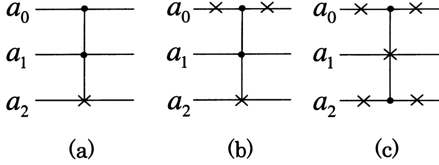
図 10: 制御 2 NOT と置換
