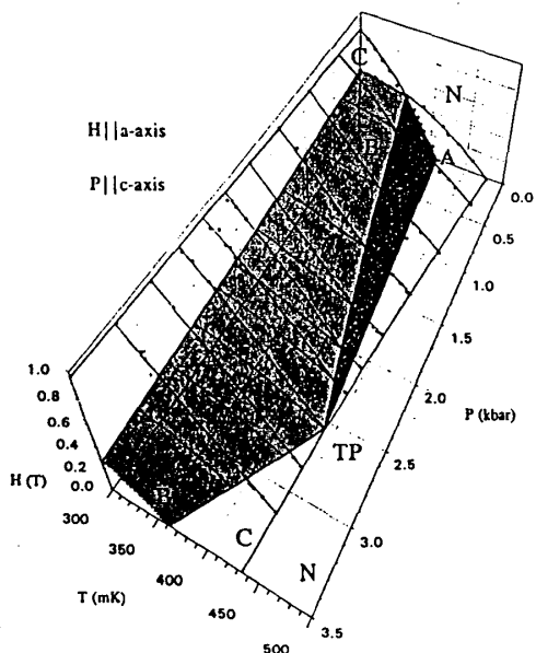
図 14: 一軸圧力下 ( P \parallel c ) の弾性測定による \text{UPt}_3 の H - T - P 相図 [38]
