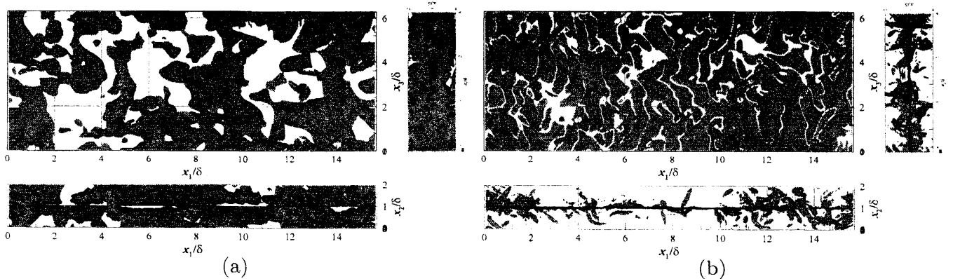
図-11 完全透過チャネル乱流における秩序構造の三面図：(a) 主流方向変動流速の等値面図（図-9(b) に対応），(b) 速度勾配テンソルの第二不変量の等値面図（図-10(b) に対応）．
