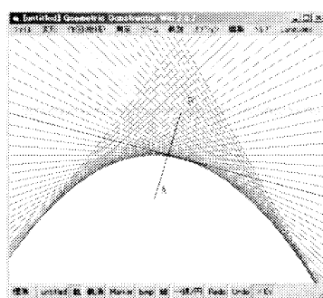
図 6 垂直二等分線の軌跡
