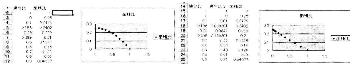
図 19 測定結果を Excel で調べる
