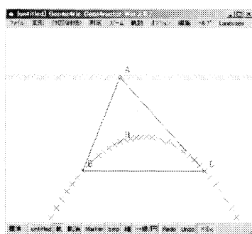
図 5 点（垂心）の軌跡
