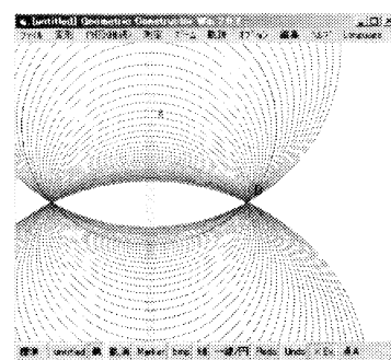
図 7 (定点を通る) 円の軌跡
