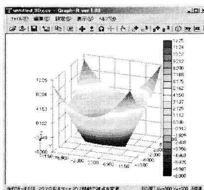
図 9 f(P) = PA + PB - 20 の様子 (3D 表示と等高線)
