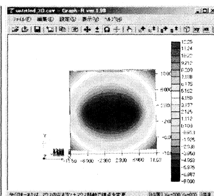
図 9 f(P) = PA + PB - 20 の様子 (3D 表示と等高線)
