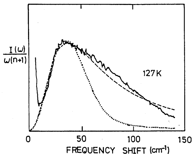
図3. プロピレングリコールのボソンピークとMBモデルの計算結果。
